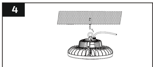
Haken sichern in dem die Mutter festgezogen wird / Secure the hook by tightening the nut
